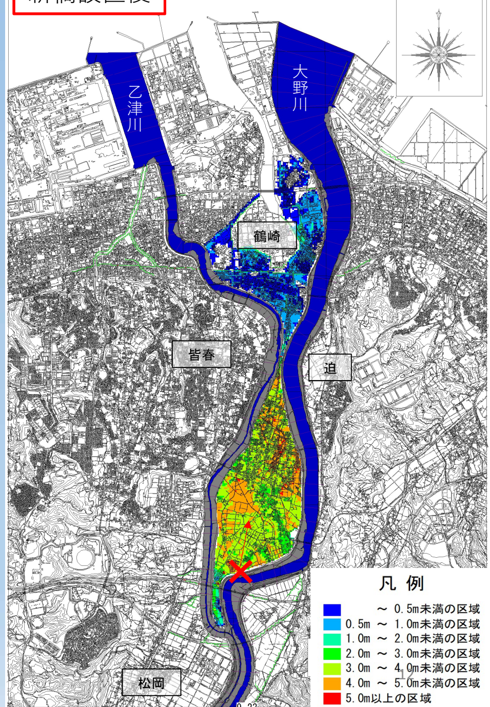
水深分布図(8.4K左岸決壊、新橋設置後)
