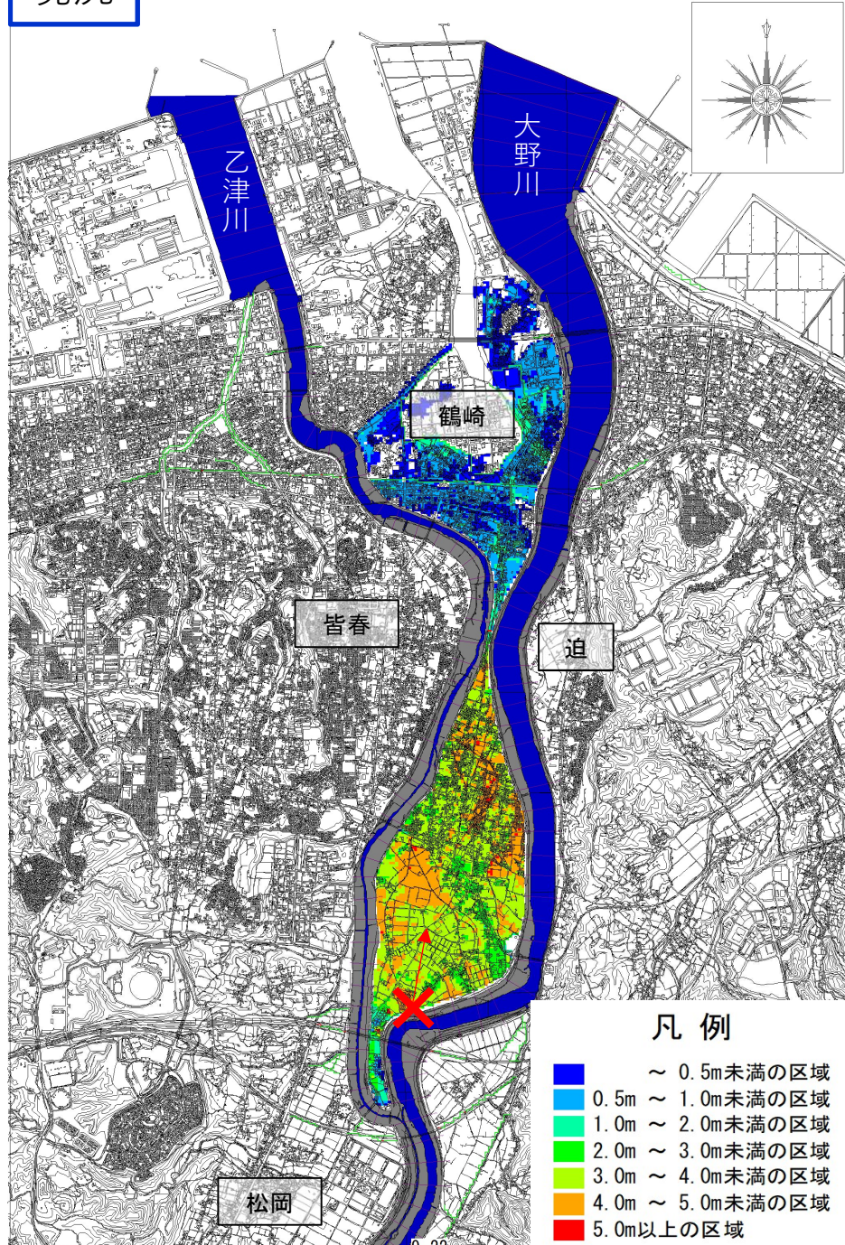
大野川浸水深分布図(8.4K左岸決壊、現況)
