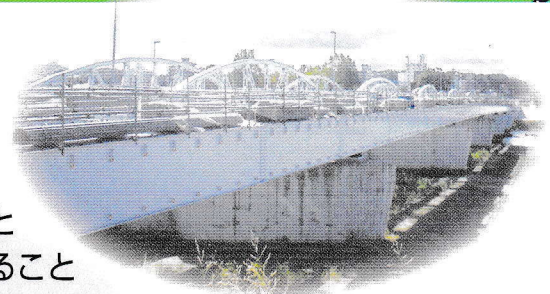
工事中の(仮称)新乙津橋(鶴崎側より)
